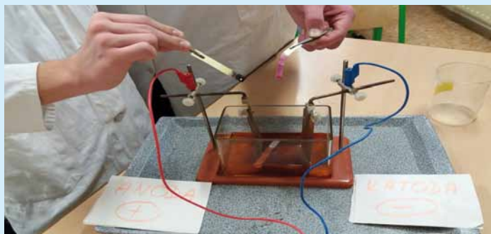
Elektrolýza roztoku jodidu draselného.
